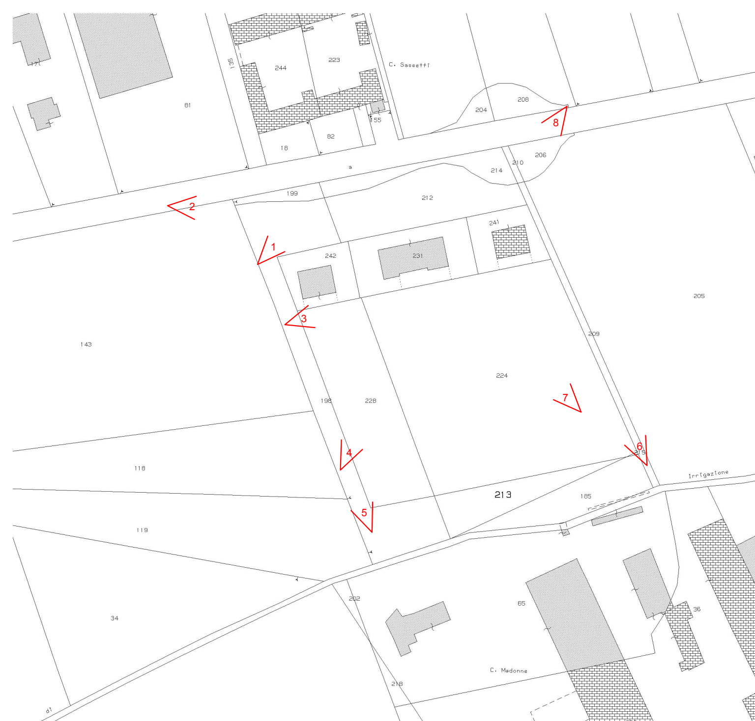
PLANIMETRIA INDIVIDUAZIONE CONI VISUALI - SCALA 1:1500
